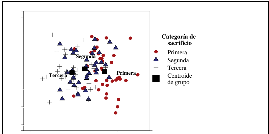
Fig. 1. Resultado de la evaluación de la pertenencia a los grupos en el análisis discriminante
